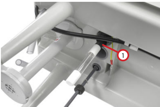
Abb. 8.1.2.7: UV-Lampe ohne Quarzglasröhre.
